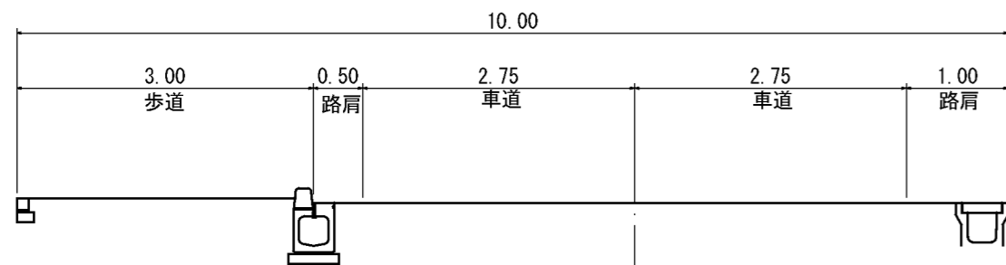
町道標準断面図
